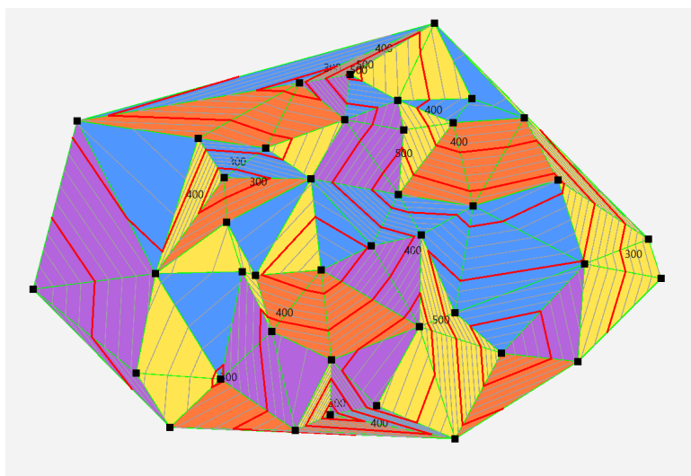
Obrázek 7.5: Expozice základních směrů, random terrain
