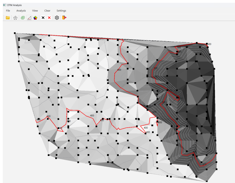
Obrázek 8.4: Vizualizace sklonu nad testovacími body
