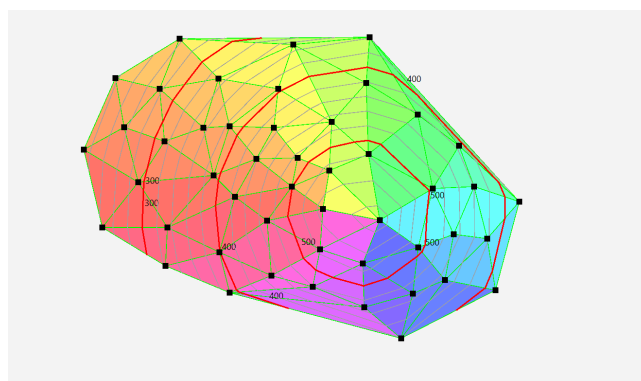
Obrázek 5.3: Vrstevnice u režimu hill
