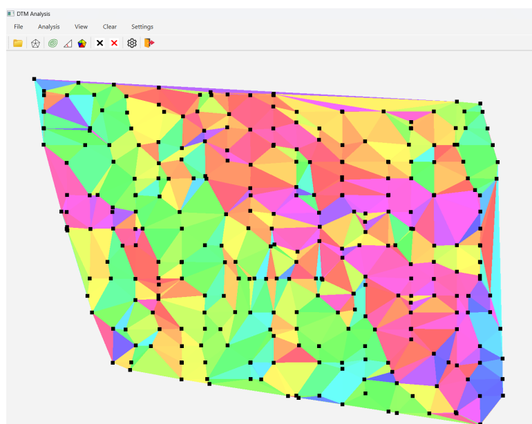
Obrázek 8.5: Vizualizace expozice nad testovacími body
