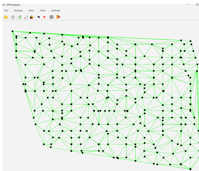
Obrázek 8.2: Vytvořená triangulace nad testovacími body
